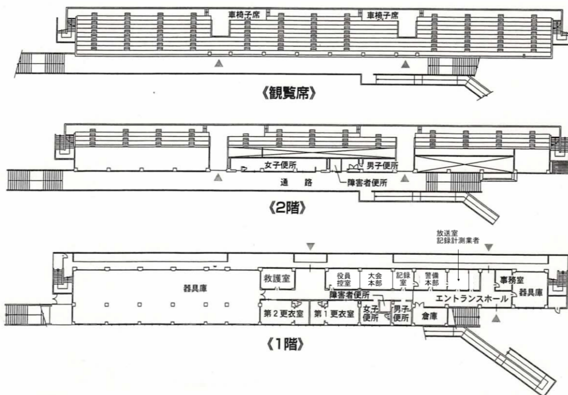
メインスタンド平面図
